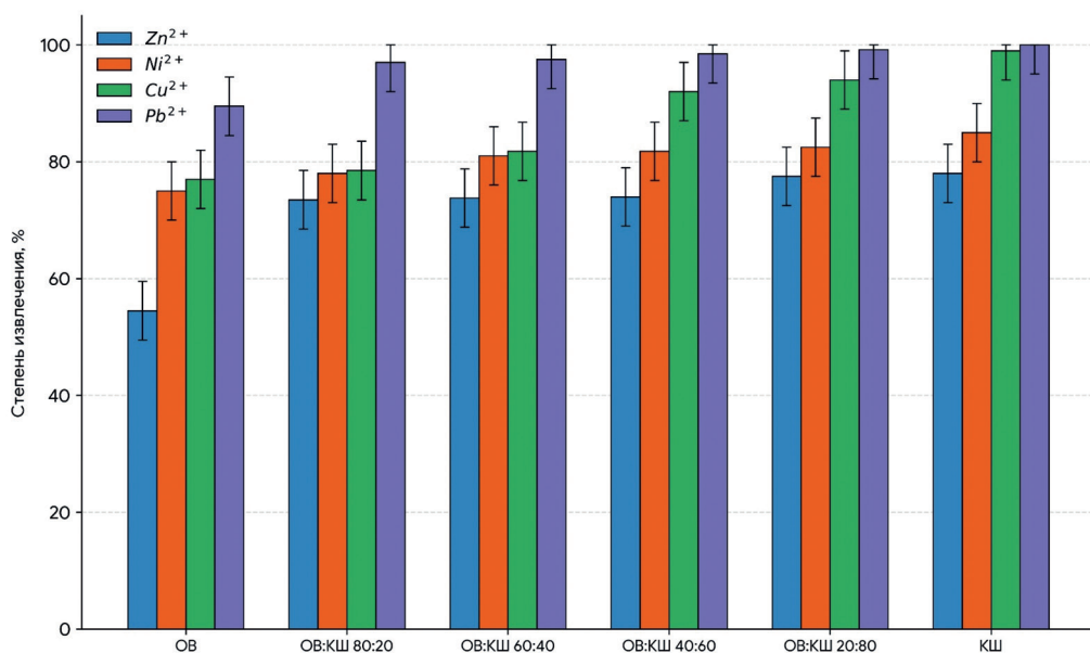
Рис. 3. Степень извлечения ионов тяжелых металлов осадками водоподготовки, красным шламом и композитными сорбентами на их основе
