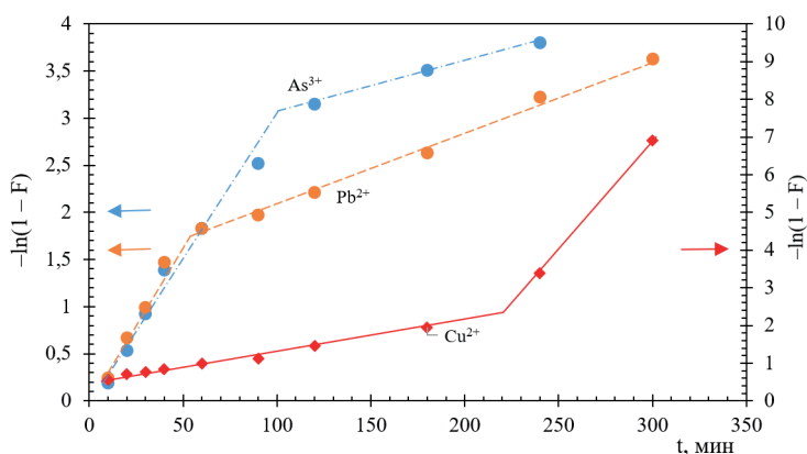
Рис. 1. Адсорбция ионов тяжелых металлов композитным сорбентом (осадки водоподготовки / торф 20 мас. %) при 298 К из растворов с исходной концентрацией 20 ПДК. Зависимость -\ln(1 - F) = f(t)
