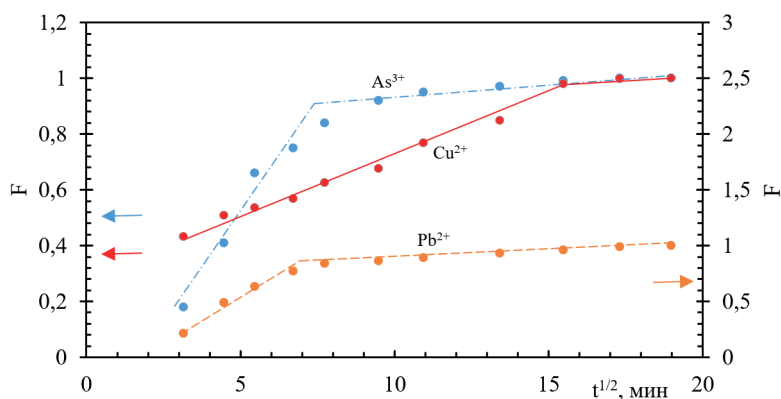
Рис. 2. Адсорбция ионов тяжелых металлов композитным сорбентом (осадки водоподготовки / торф 20 мас. %) при 298 К из растворов с исходной концентрацией 20 ПДК. Зависимость F = f(t^{1/2})
