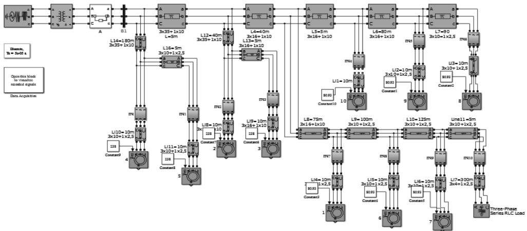
Рис. 1. Моделирование сети шахты с преобразователями частот
