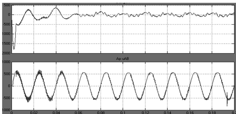
Рис. 2. Форма волны тока и напряжения в фазе А
