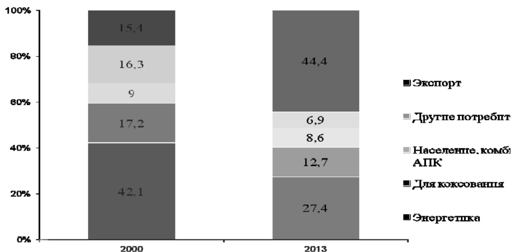
Рис. 2. Структура поставок российского угля в 2000 и 2013 гг., %
