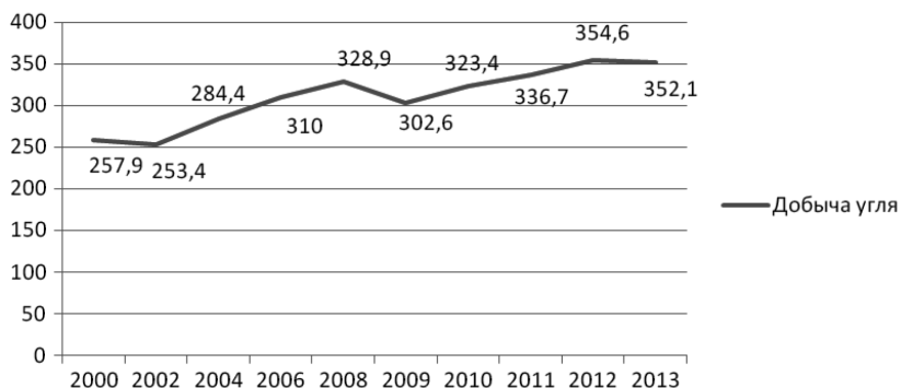
Рис. 1. Добыча угля в России (в млн т)
