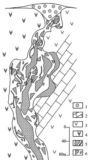
Рис. 2. Черемшанская залежь Уфалейского месторождения: 1 – нерудносные кремнистые охры; 2 – известняки; 3 – серпентиниты; 4 – серпентиниты гидратированные, иногда рудоносные; 5 – руды никелевых силикатов и кварца, иногда ожелезненные желваковые и линзовидные (Ni 3–5%, иногда до 10–15%); 6 – серпентинитовый приразломный меланж с гидросиликатами никеля (Ni 0,9–2%)
