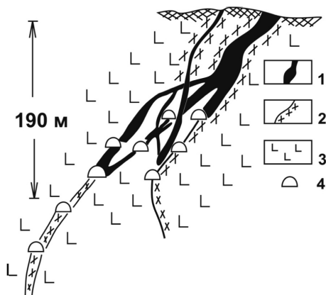
Рис. 3. Разрез оработанного месторождения Боа-Кфин, Новая Гвинея (по Е.Гласе, Вершинину и др., 1988): 1 — рудные тела; 2 — серпентиниты окремненные; 3 — серпентиниты свежие; 4 — эксплуатационные горизонты
