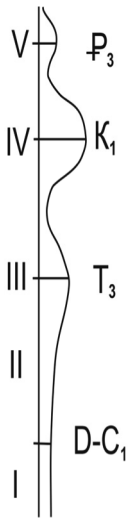
Рис. 1. Относительная интенсивность проявления рудогенерирующих процессов формирования никелевых месторождений на Урале. Эндогенная группа: I – сингенетичные сульфидные руды; II – эпигенетичные сульфидные руды. Гипергенная группа: III – оксидные руды термального гипергенеза; IV – оксидные элювиальные руды (кор выветривания и рудных шляп); V – сульфидные осадочные и осадочно-инфильтрационные рудогенерирующие процессы
